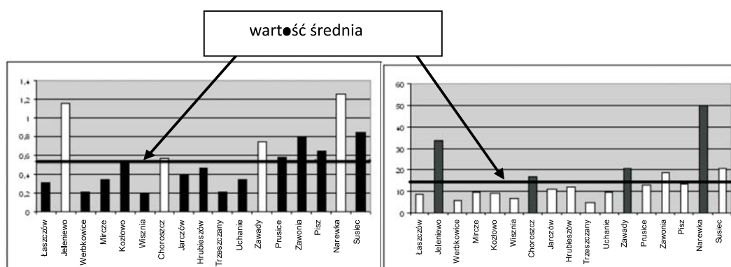
Rys. 7. Zużycie biomasy drzewnej w analizowanych gminach w odniesieniu do 1 m 2 powierzchni budynków oraz w odniesieniu do 1 osoby, w GJ/m 2 /rok oraz TJ/os/ro
