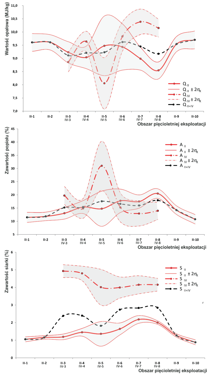
Rys. 3. Średnie wartości opałowe węgla ( Q_{lr} ), zawartości siarki ( S^d ) i popiołu ( A^d ) w węglu w granicach pięcioletnich postępów eksploatacji w pokładach II i IV oraz łącznie dla obydwu pokładów wraz zakresem prognozowanego błędu kriginu 2sK (dla prawdopodobieństwa P = 95\% )
